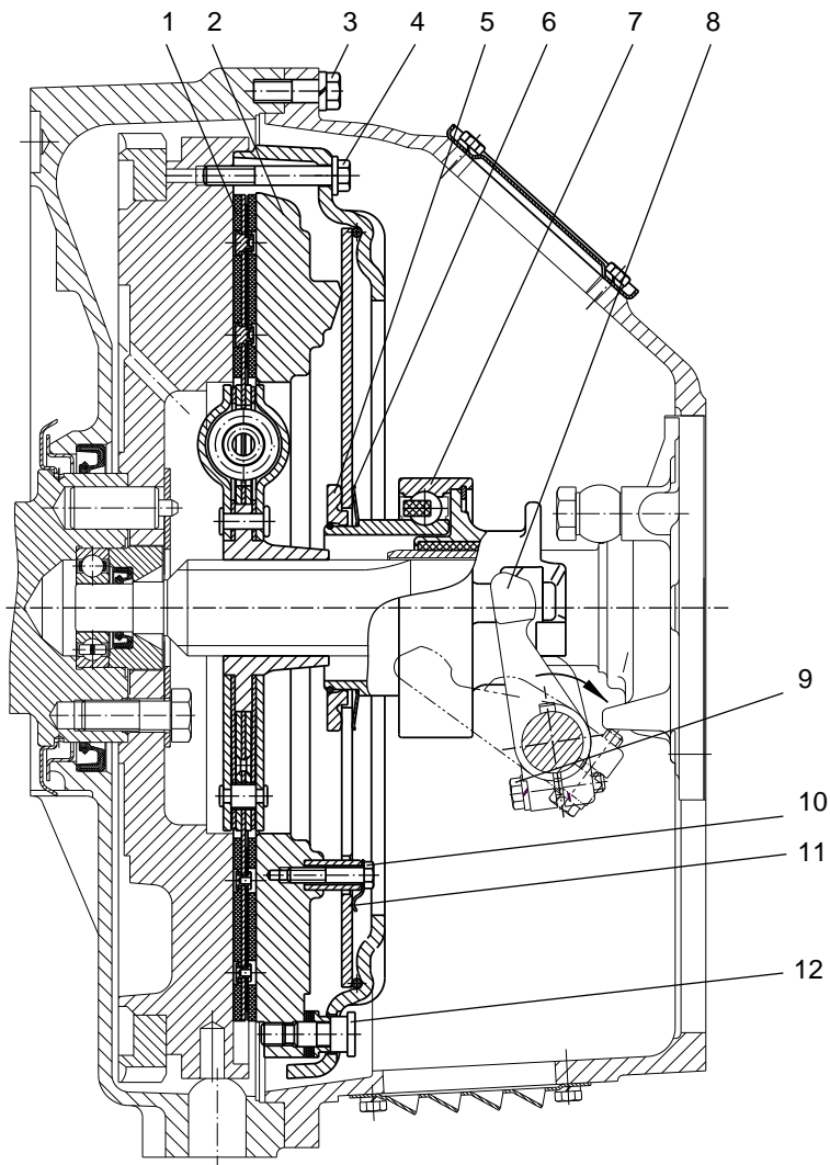
Рисунок – 24 – Сцепление:
