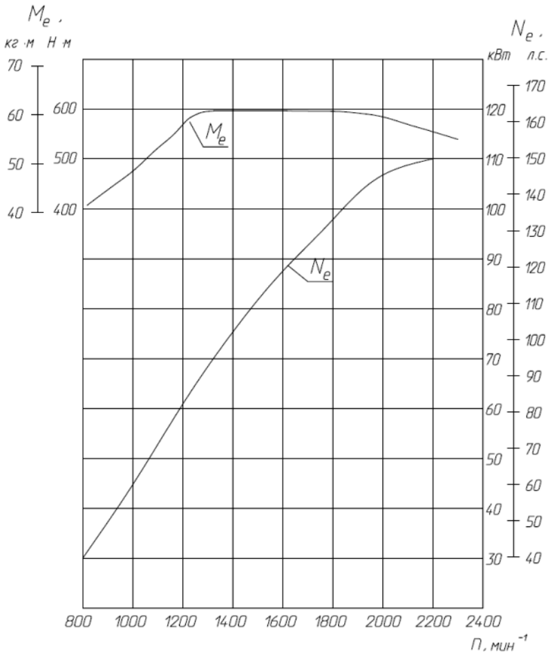
Рисунок 2а – Скоростная характеристика двигателя ЯМЗ-53424
