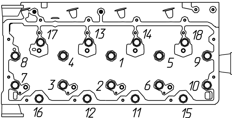
Рисунок А.1 - Порядок затяжки болтов крепления головки блока цилиндров.
